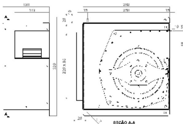
MGS 160 SIMPLES ASPIRAÇÃO COM GABINETE
