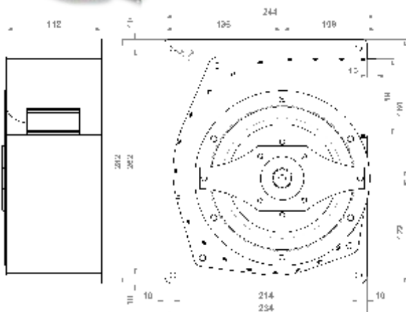
MVS 160 SIMPLES ASPIRAÇÃO
